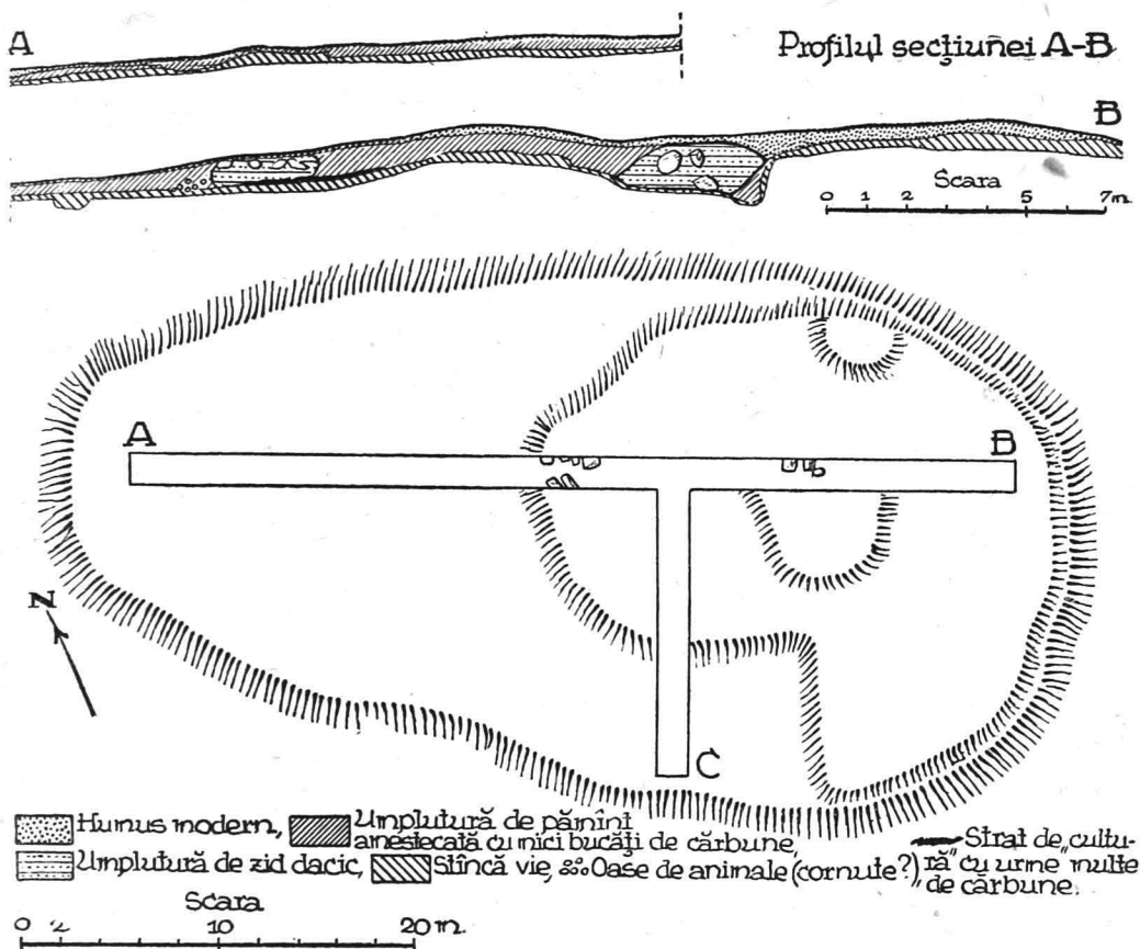
Fig. 29. — Cetățuia Înaltă. Planul general al platoului.
