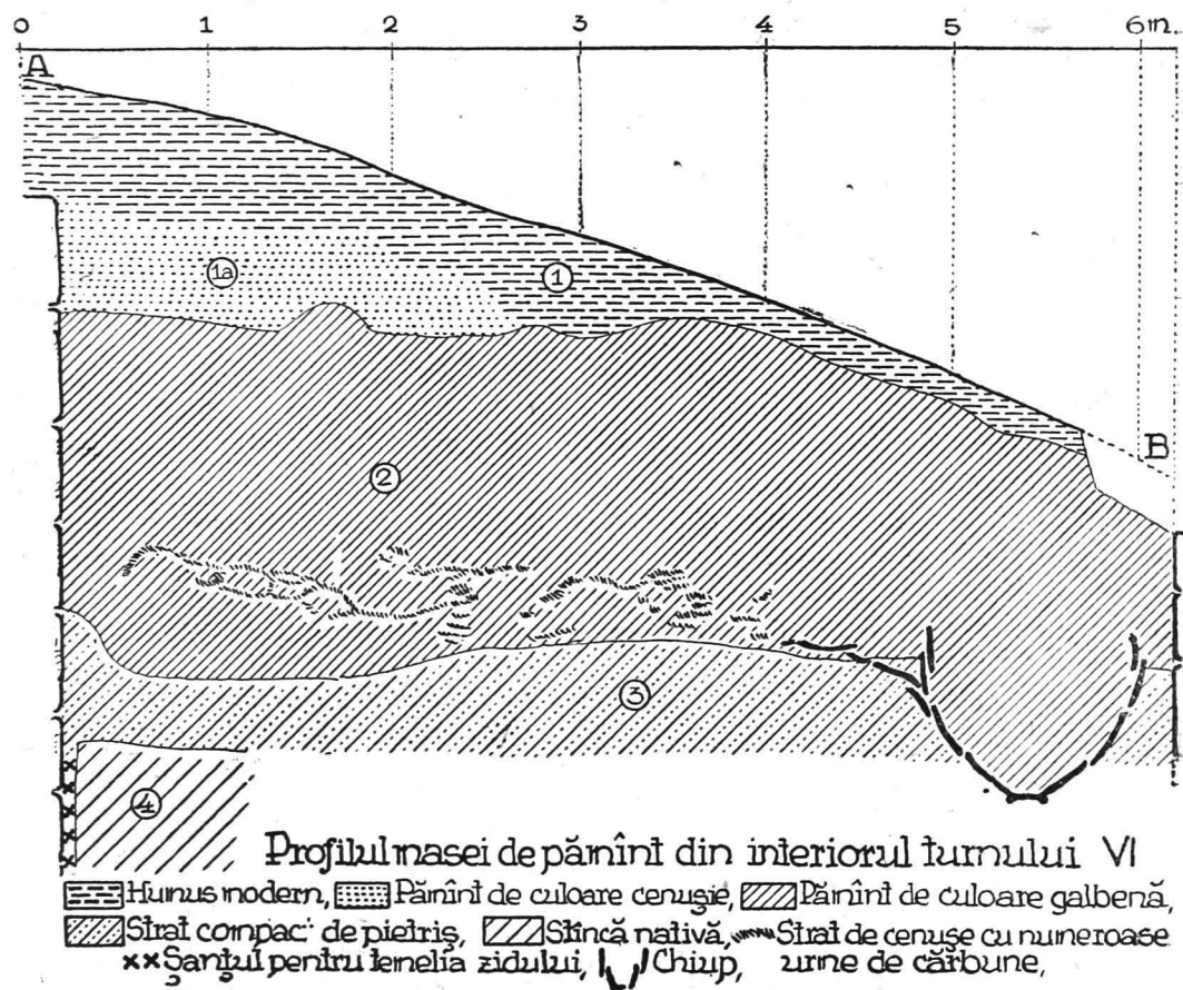
Fig. 24. — Blidarul. Profil în interiorul Turnului VI.
