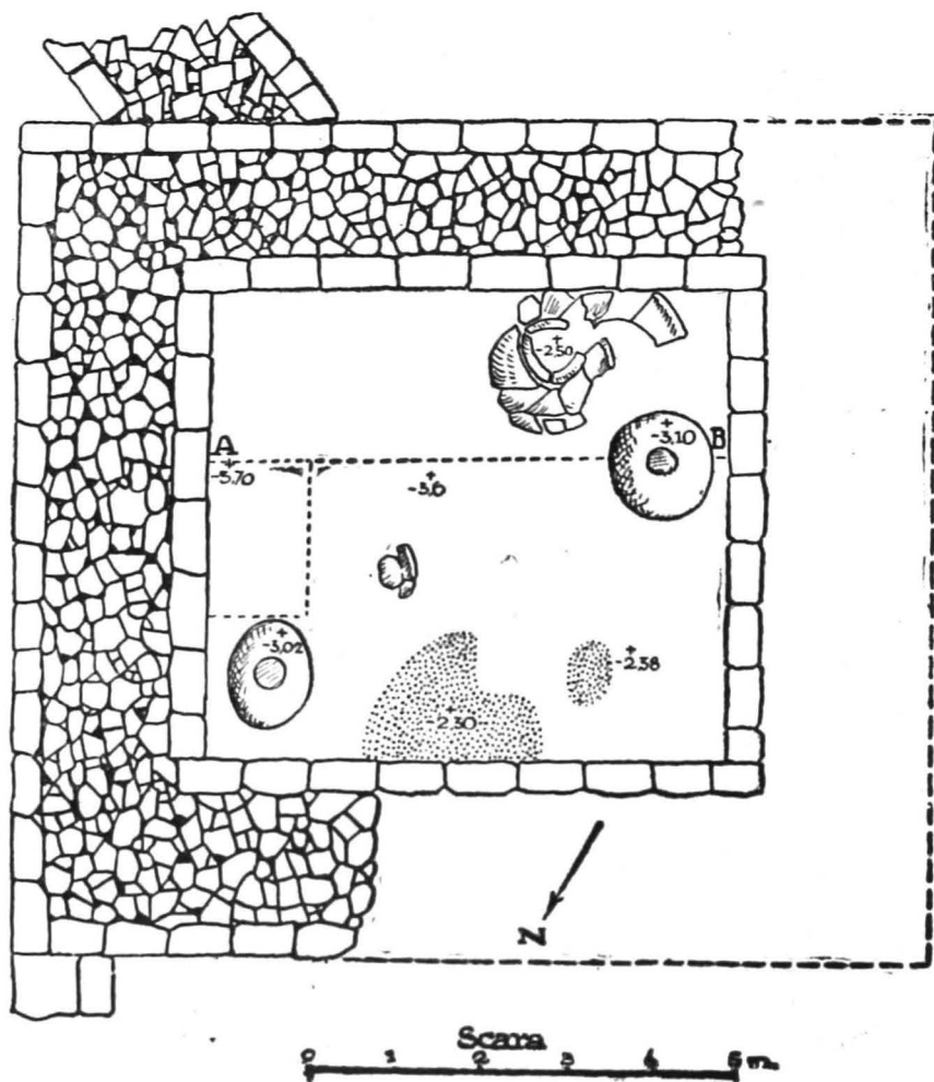
Fig. 23. — Blidarul. Planul Turnului VI.
