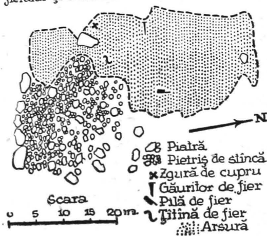
Fig. 15. — Grădiștea Muncelului. Atelierul. Cuptorul nr. III.
