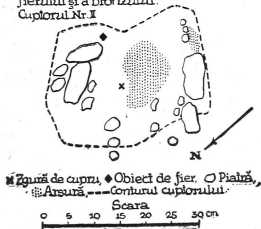
Fig. 14. — Grădiștea Muncelului. Atelierul. Cuptorul nr. II.
